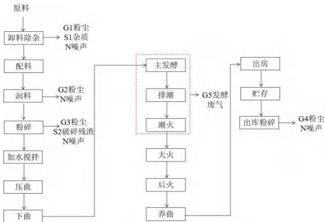
图 3-6 生产工艺流程图及产污环节图
