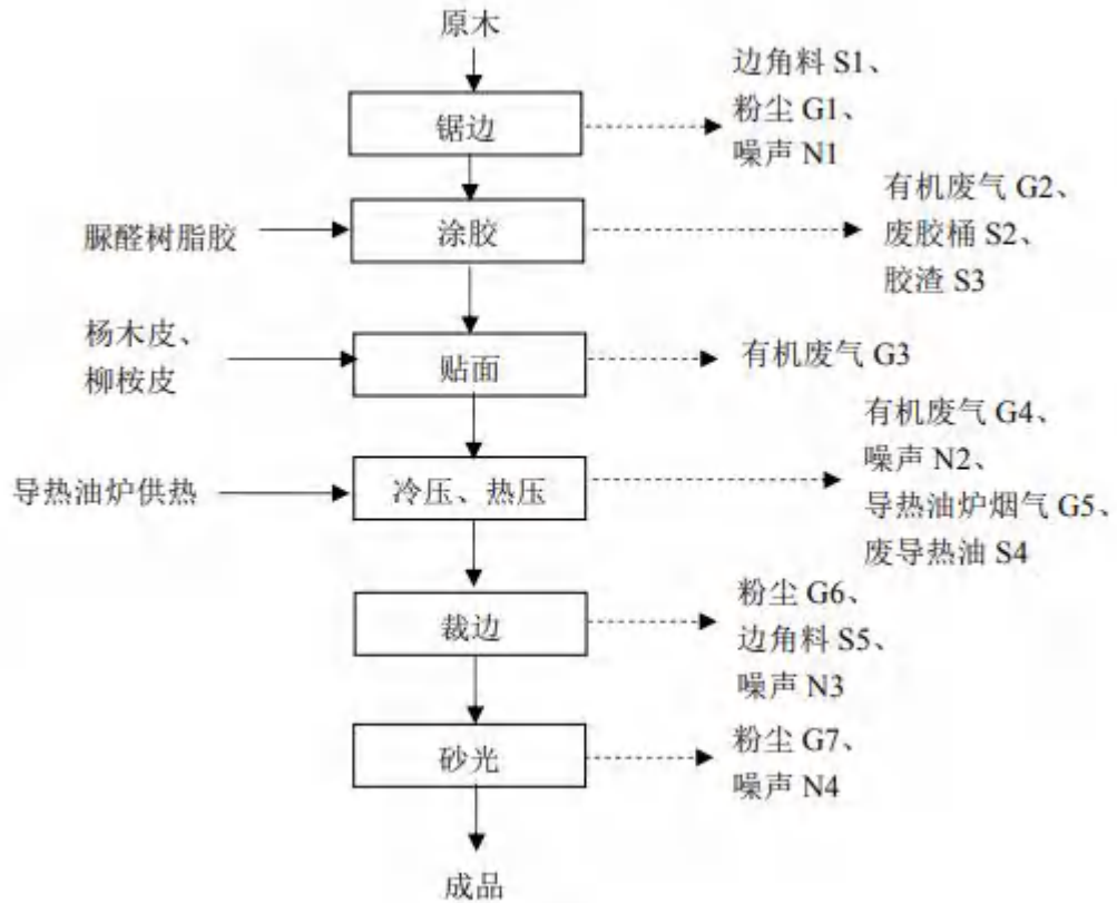
图 2-2 细木工板生产工艺流程及产污环节图
