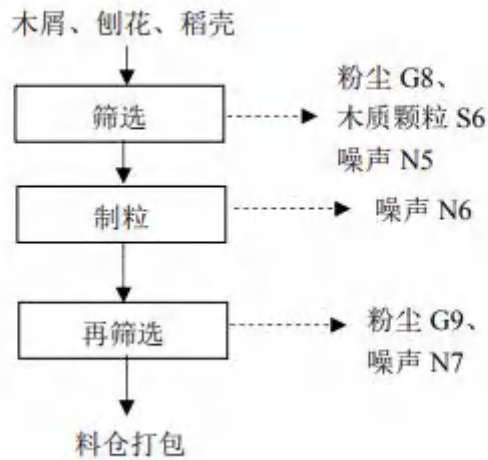
图2-3 木质生物燃料生产工艺流程及产污环节图
